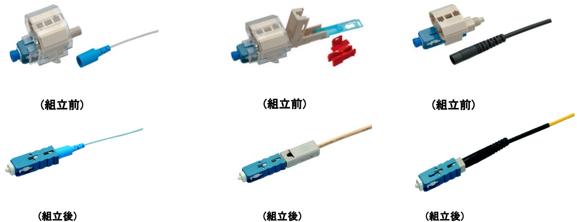
FAST—SCコネクタ 0.25mm素線及び 0.9mm心線用
